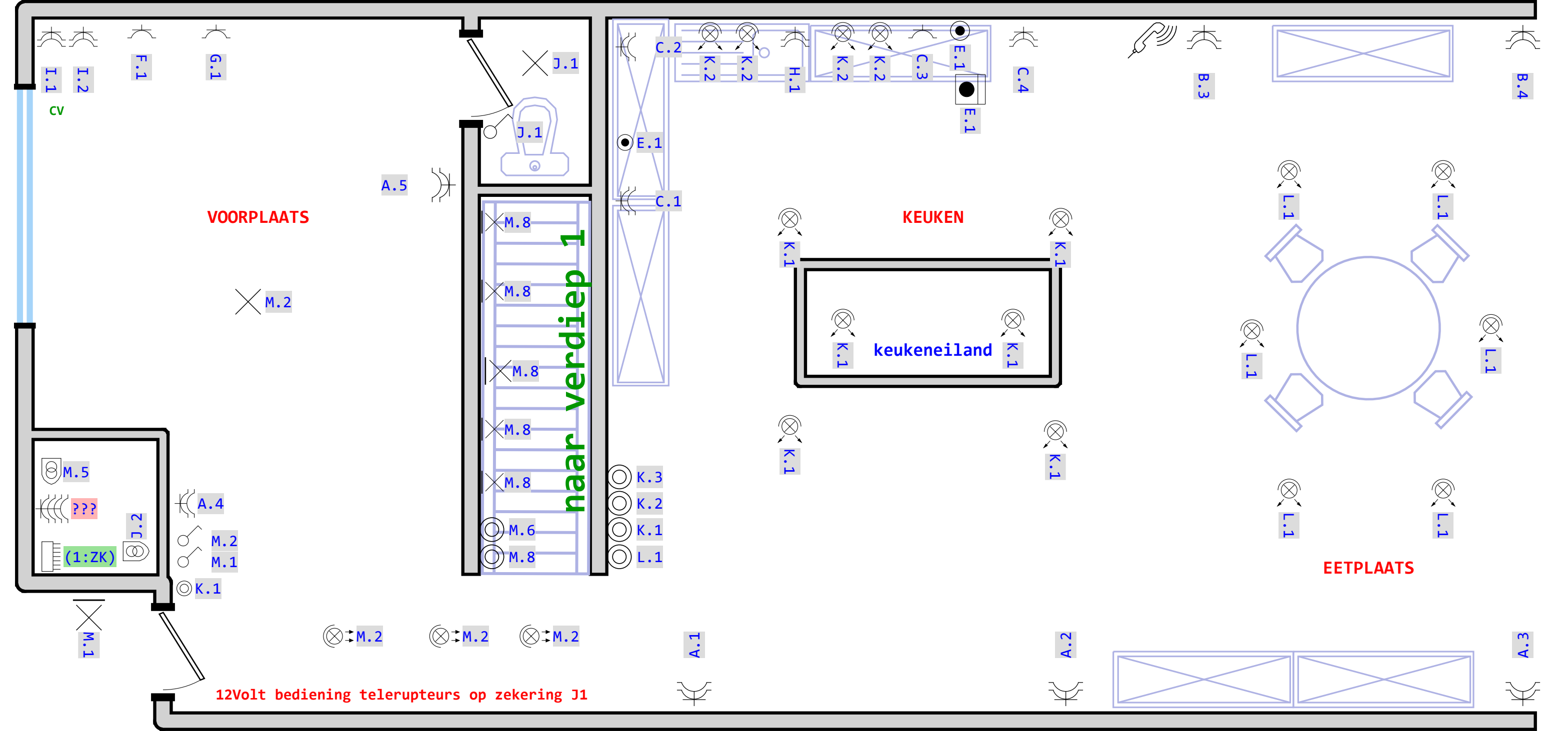
VERDIEP 0
